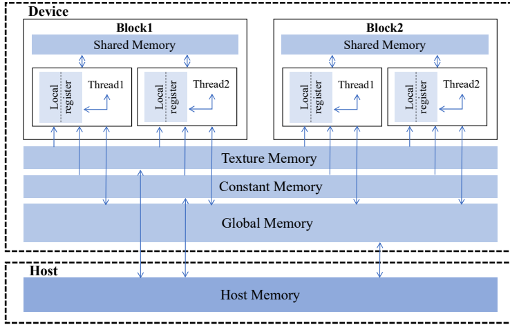
Fig. 1. Memory Hierarchy [28]
